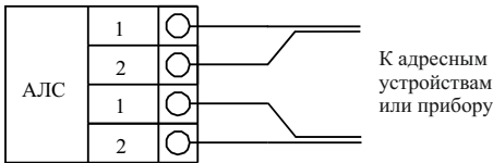
Рисунок 2 – Схема подключения
