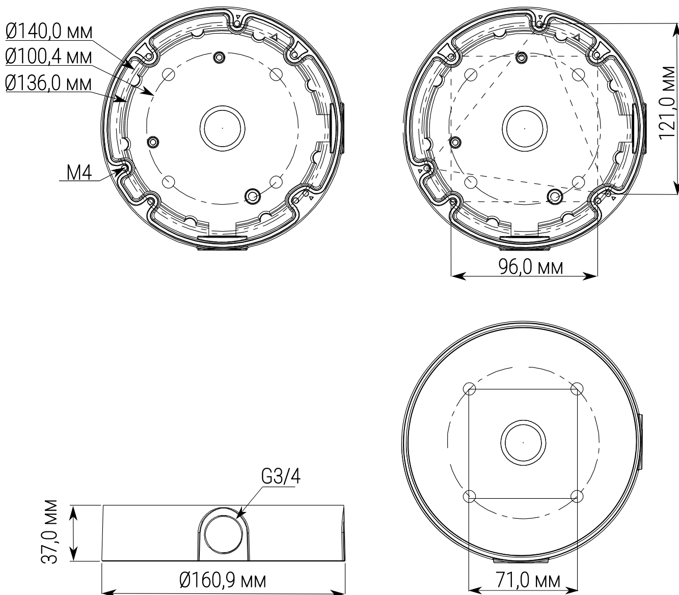
Рисунок 4.1 – Габаритные размеры
