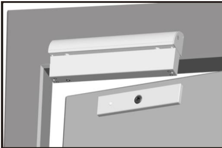
Рис.1 «Установка LC-крепления»
