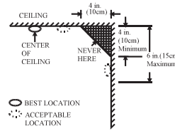
Рисунок 4: РЕКОМЕНДУЕМЫЕ ЛУЧШИЕ И ПРИЕМЛЕМЫЕ МЕСТА УСТАНОВКИ ДЫМОВОГО ДАТЧИКА
